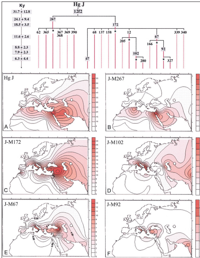
Εικ. 1. A-G: Φυλογένεση και κατανομή των συχνοτήτων της απλοομάδας J του χρωμοσώματος Y, καθώς επίσης βασικών γενεαλογικών γραμμών της σε σύγχρονους Ευρασιατικούς και Αφρικανικούς πληθυσμούς ανθρώπων. Στο πάνω αριστερό μέρος του φυλογενετικού δένδρου δίνεται η μέση ηλικία (σε χιλιάδες χρόνια) αρχικής δημιουργίας των μεταλλάξεων (εντός παραλληλογράμμων) συν το τυπικό σφάλμα 12 .
